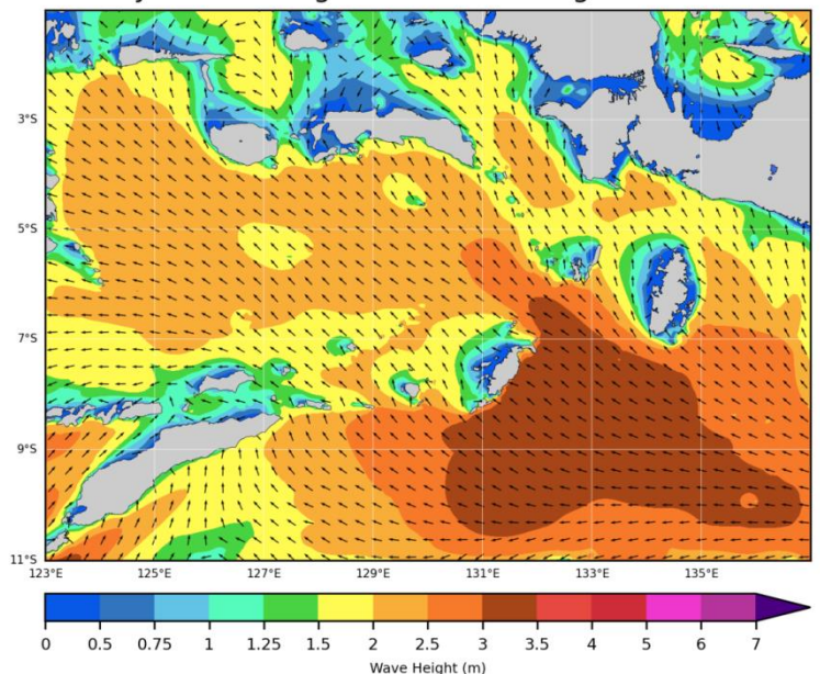
Gambar 3.14 Gelombang Signifikan Tertinggi Absolut bulan Oktober 2020 (Sumber : BMKG Pusat)
