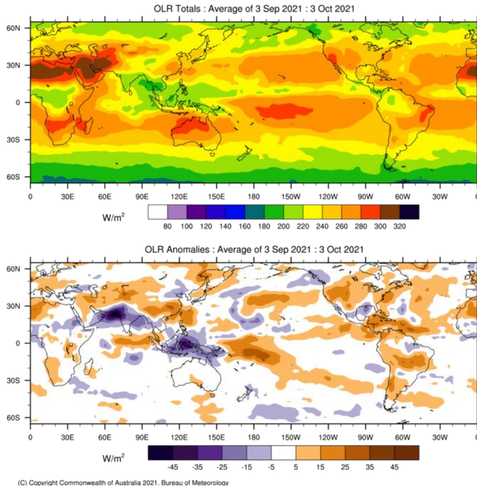
Gambar Total dan Anomali OLR (Sumber : http://www.bom.gov.au )
