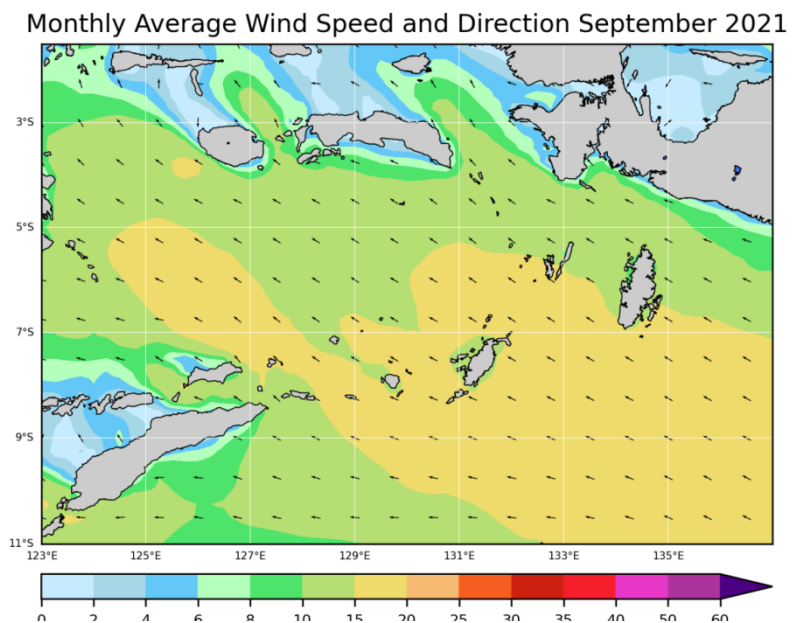
Gambar Arah dan Kecepatan Angin Rata-Rata bulan September 2021
