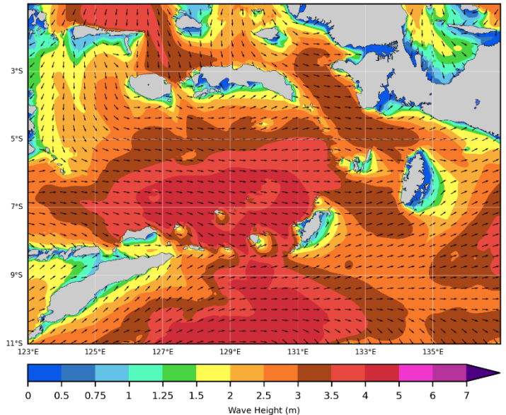
Gambar Gelombang Signifikan Tertinggi Absolut bulan Februari 2022 (Sumber : BMKG Pusat)
