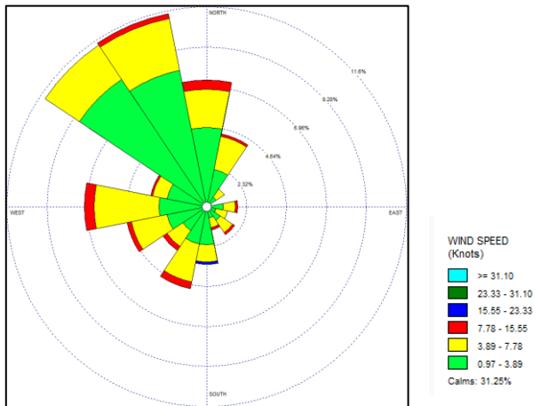
Gambar Windrose angin permukaan bulan Januari 2023
