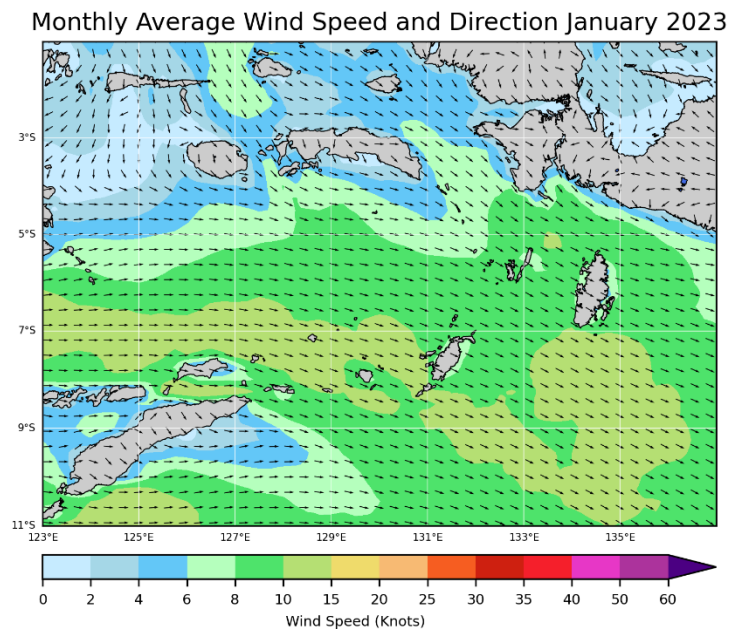
Gambar Arah dan Kecepatan Angin Rata-Rata Bulan Januari 2023 (Sumber : BMKG Pusat)
