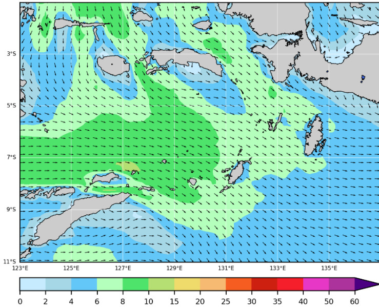
Gambar Arah dan Kecepatan Angin Rata-Rata bulan Februari 2022 (Sumber : BMKG Pusat)
