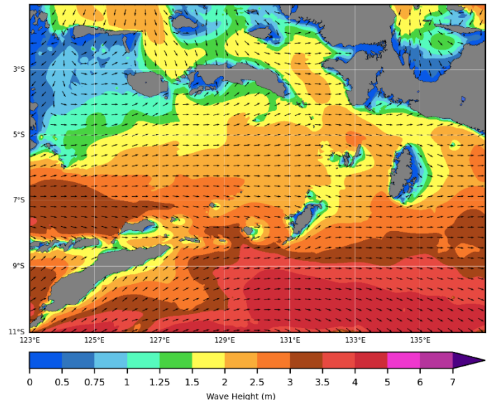
Gambar Gelombang Signifikan Tertinggi Absolut Bulan Januari 2023 (Sumber : BMKG Pusat)
