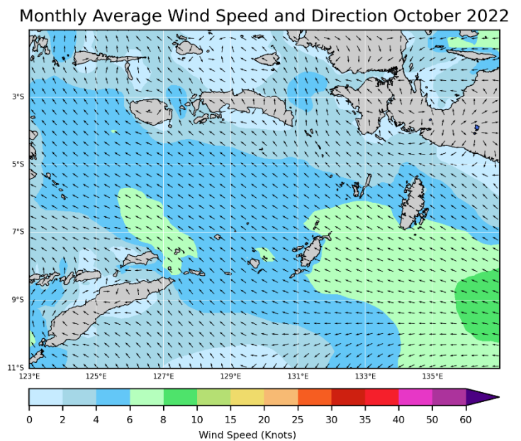
Gambar Arah dan Kecepatan Angin Rata-Rata Bulan Oktober 2022 (Sumber : BMKG Pusat)
