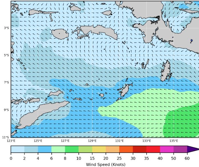
Gambar Arah dan Kecepatan Angin Rata-Rata bulan November 2021 (Sumber : BMKG Pusat)
