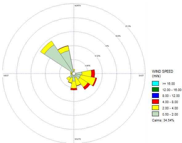
Gambar Windrose angin permukaan bulan Oktober 2022
