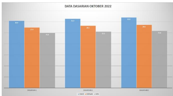
Gambar Suhu rata - rata bulan Oktober 2022
