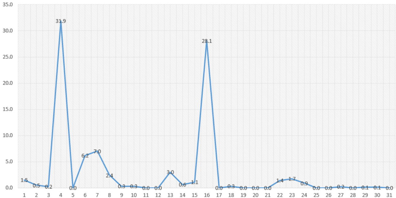
Gambar Curah hujan Harian bulan Oktober 2022
