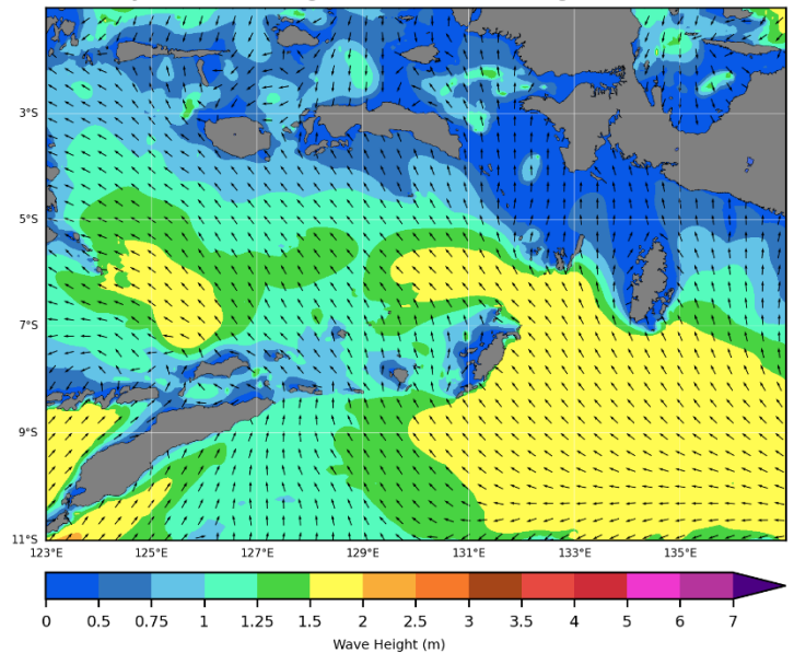
Gambar Gelombang Signifikan Tertinggi Absolut Bulan Oktober 2022 (Sumber : BMKG Pusat)
