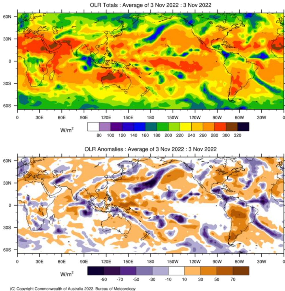
Gambar Total dan Anomali OLR (Sumber : http://www.bom.gov.au )
